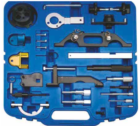
Motor-Steuerzeiten
